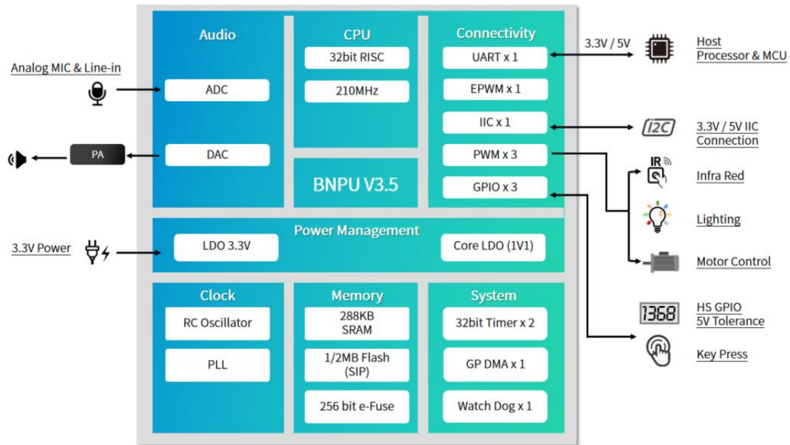
图 1-1 CI13082V 功能框图
