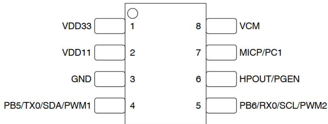
图 2-1 CI13082V 管脚顺序及定义图
