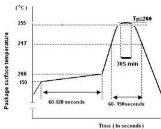
图 6-2 炉温曲线图
